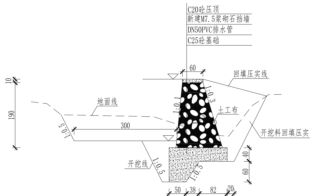
图 4-2 排洪沟标准断面图
