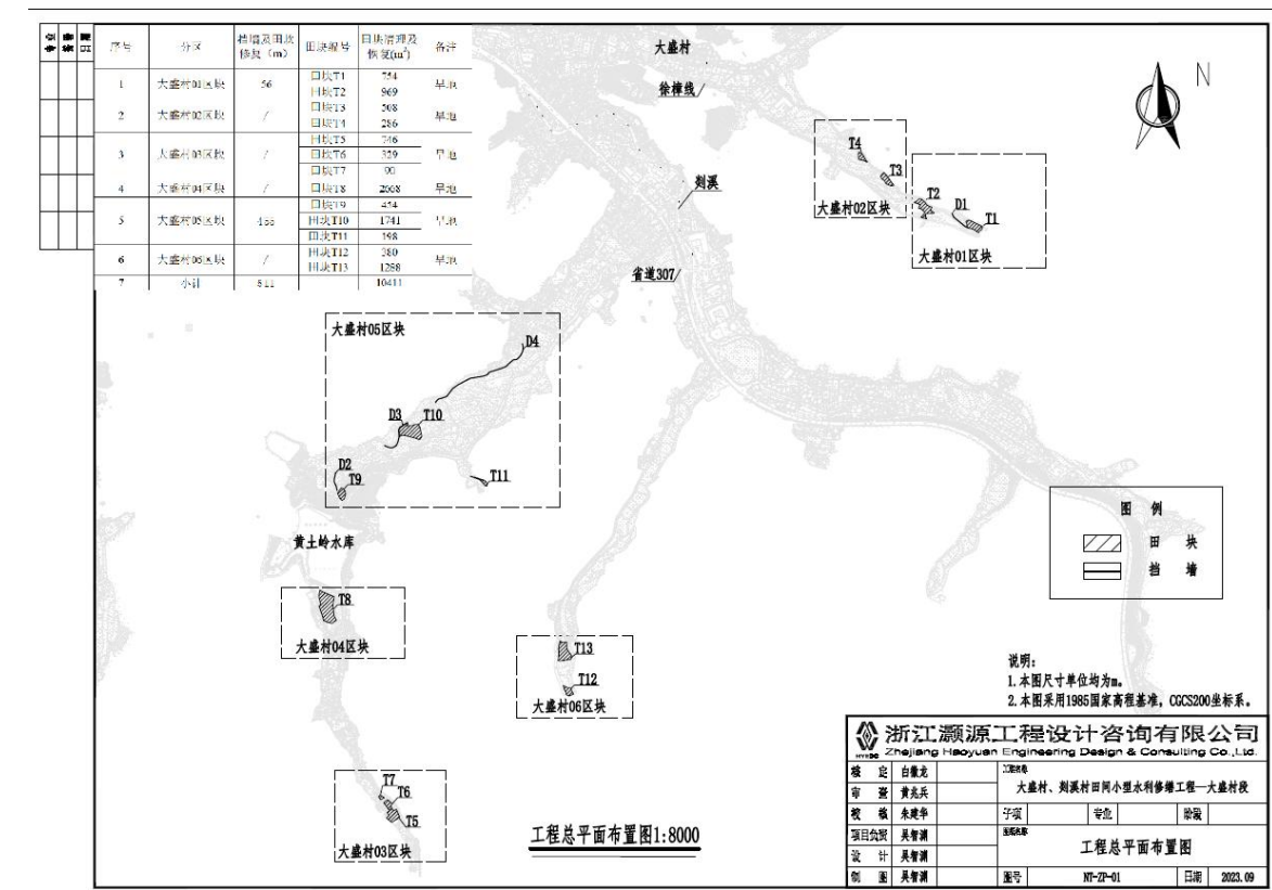
图 4-1 大盛村、剡溪村总平面布置图
