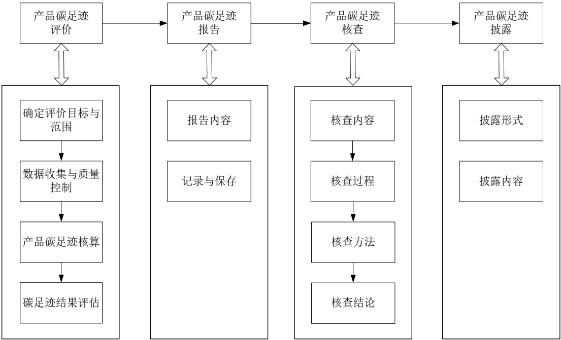
图1 产品碳足迹评价工作流程图示
