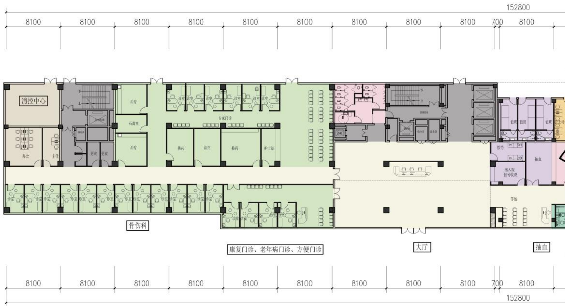
一层西区平面
