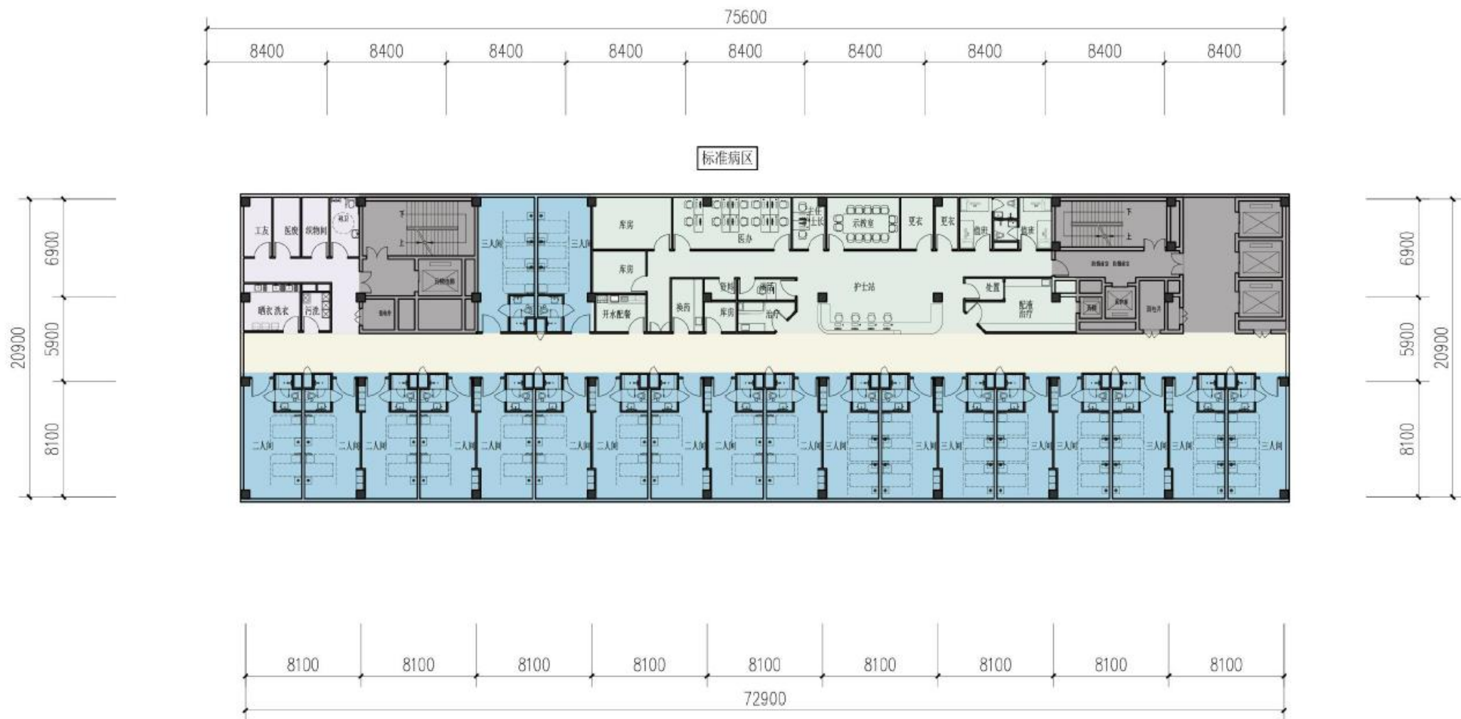
七-八层平面
